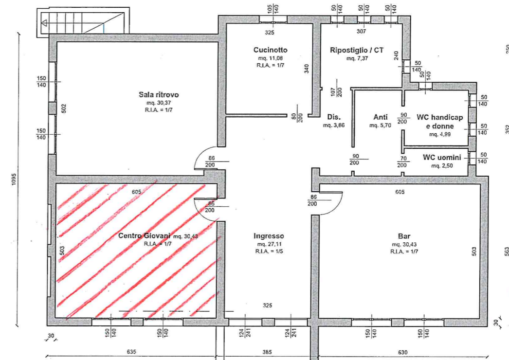
PIANTA TERRA
