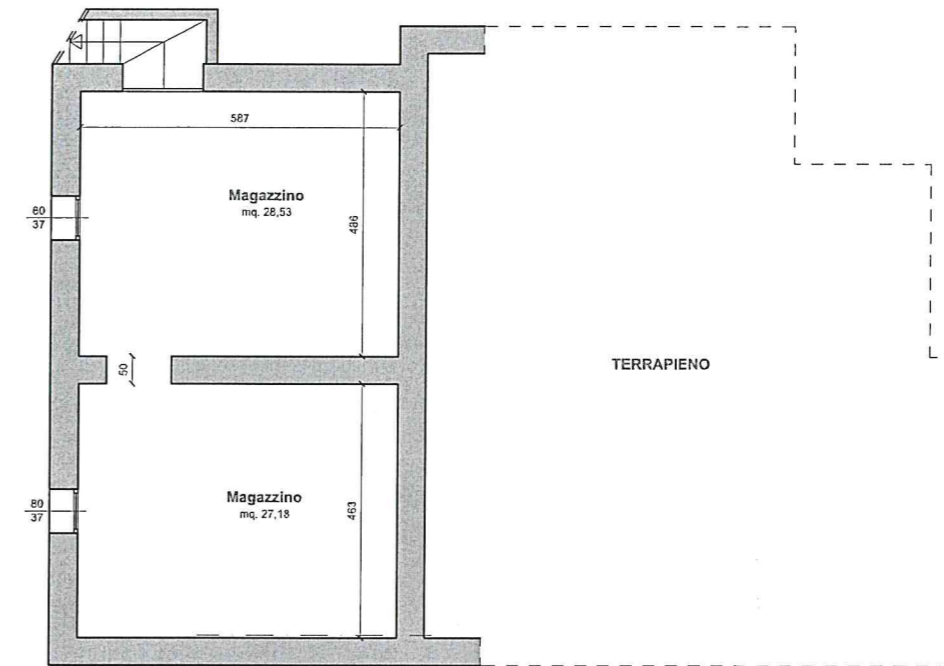
PIANTA SOTTOSTRADA
